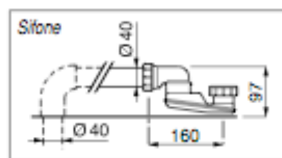
Particolare dello scarico. Detail of drain
